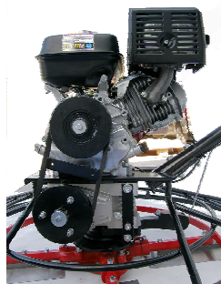
Widok sprzęgła odśrodkowego po zdjęciu osłony
